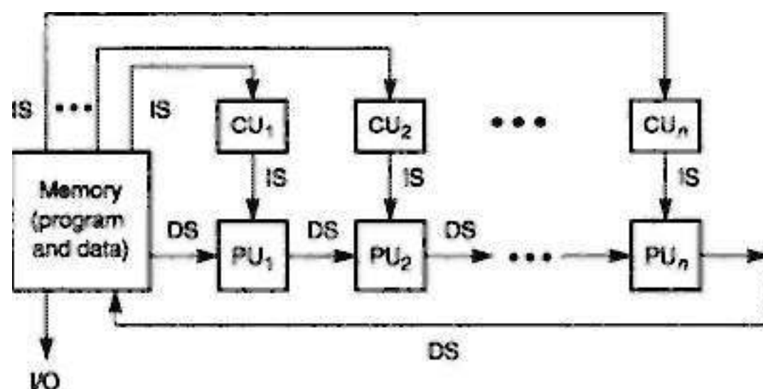
(d) MISD architecture (the systolic array)
